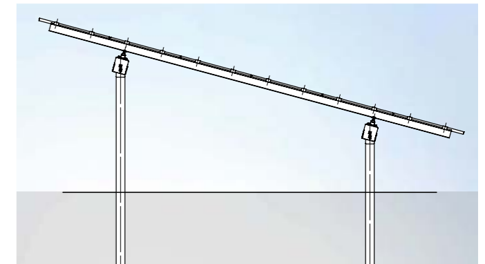
Schematische Darstellung Modultisch Bereich B
